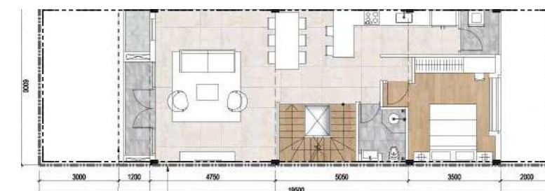
Mặt Bằng Tầng 2 | 2 nd Floor
