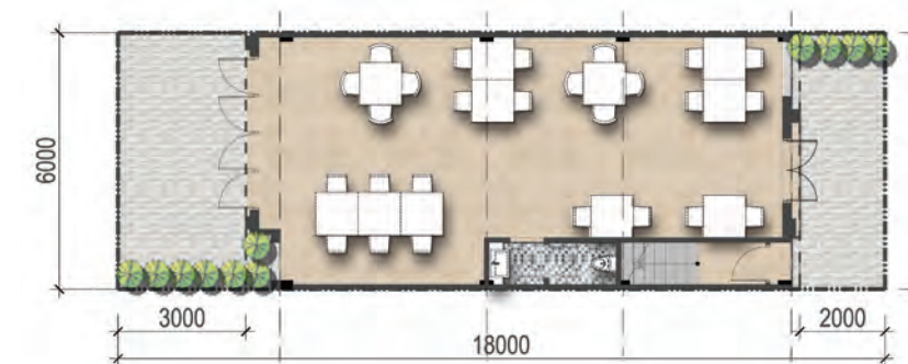
Mặt Bằng Tầng 1 | 1 st Floor
