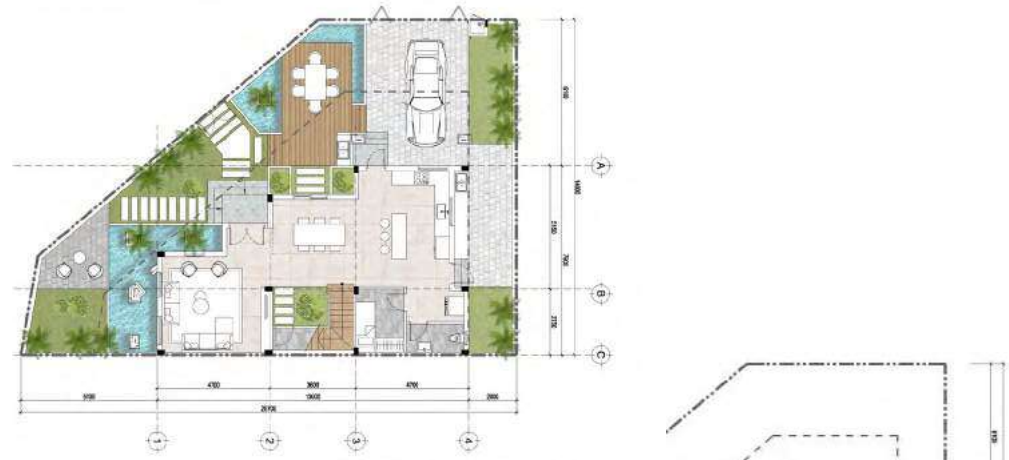
Mặt Bằng Tầng 1 | 1 st Floor
