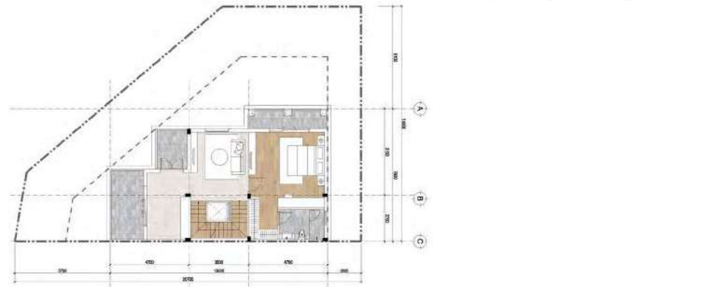
Mặt Bằng Tầng 3 | 3 rd Floor
