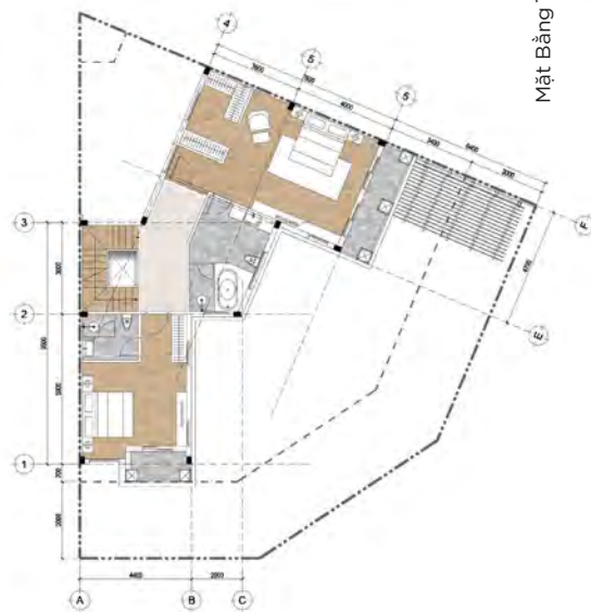
Mặt Bằng Tầng 2 | 2 nd Floor
