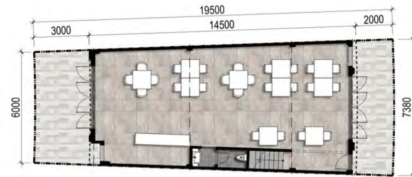
Mặt Bằng Tầng 1 | 1 st Floor
