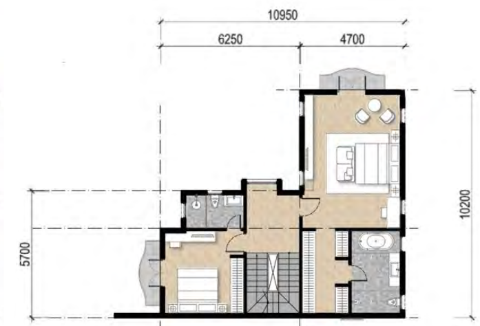
Mặt Bằng Tầng 3 | 3 rd Floor
