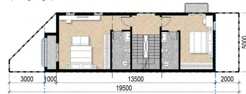
Mặt Bằng Tầng 2 | 2 nd Floor
