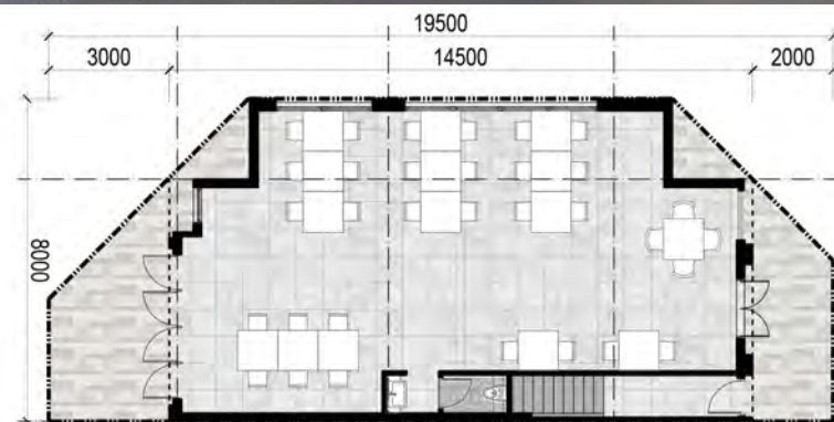
Mặt Bằng Tầng 1 | 1 st Floor
