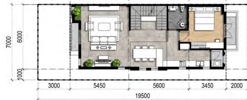
Mặt Bằng Tầng 2 | 2 nd Floor
