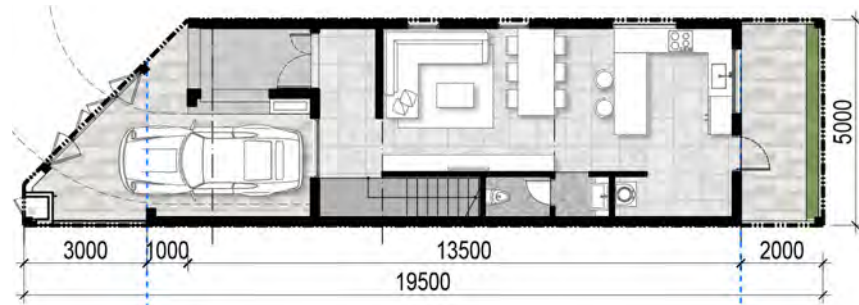
Mặt Bằng Tầng 1 | 1 st Floor
