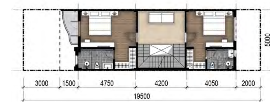
Mặt Bằng Tầng 2 | 2 nd Floor
