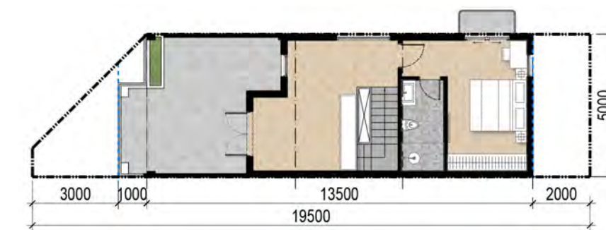
Mặt Bằng Tầng 3 | 3 rd Floor
