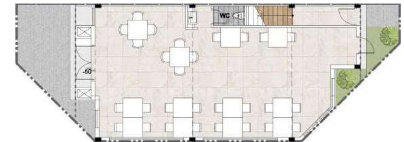
Mặt Bằng Tầng 1 | 1 st Floor
