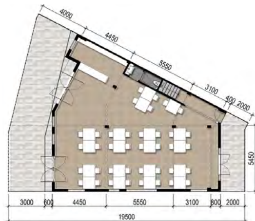
Mặt Bằng Tầng 1 | 1 st Floor
