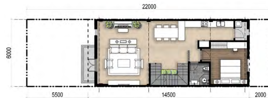
Mặt Bằng Tầng 2 | 2 nd Floor
