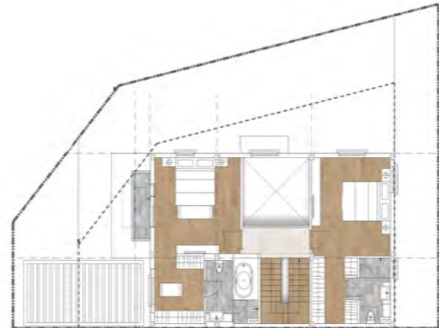
Mặt Bằng Tầng 2 | 2 nd Floor
